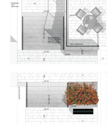
Ul. Kręta. Detal posadzki 1:50
