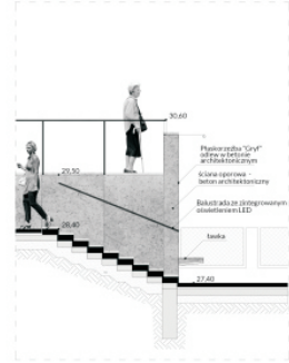
Ul. Kręta. Szczegół b-b 1:50
